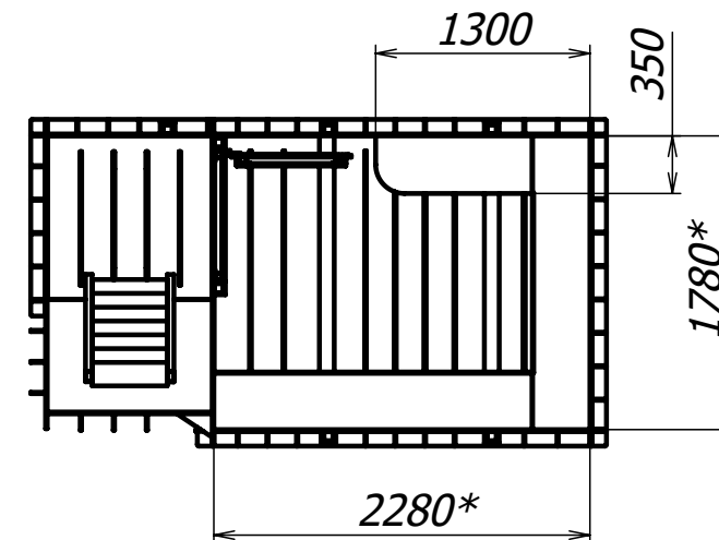
Г-Г (1 : 50)
