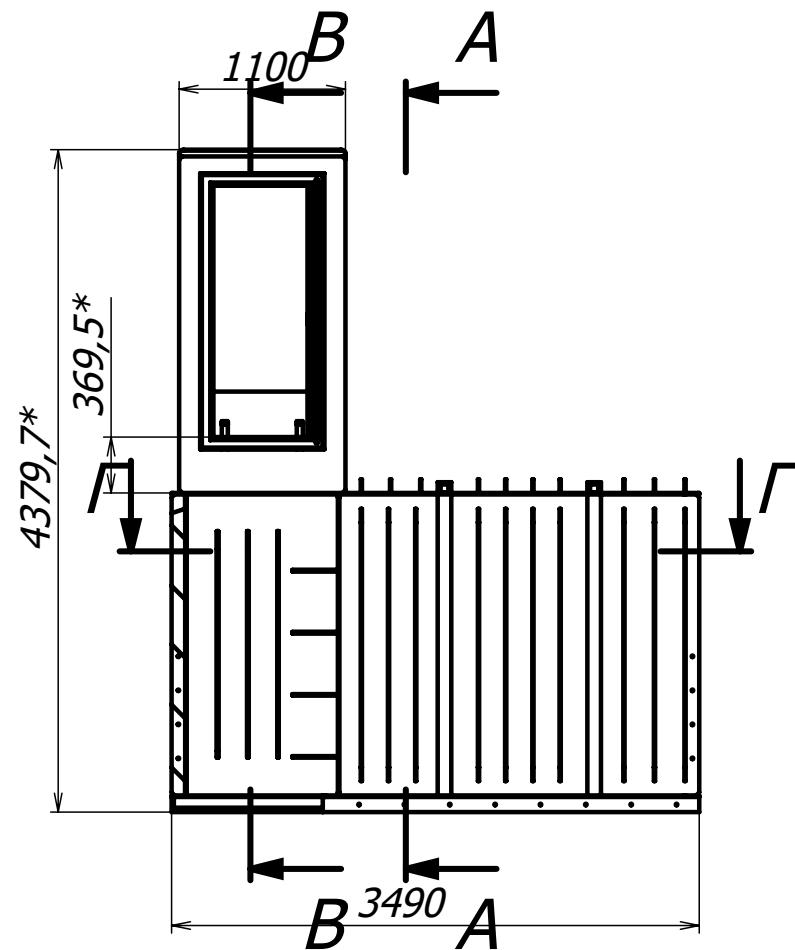
В-В (1 : 50)
