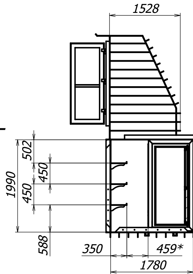
Г-Г (1 : 50)
