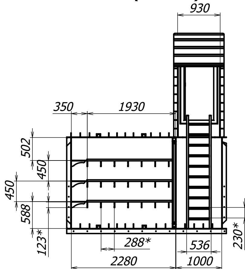
Б-Б (1 : 50)
